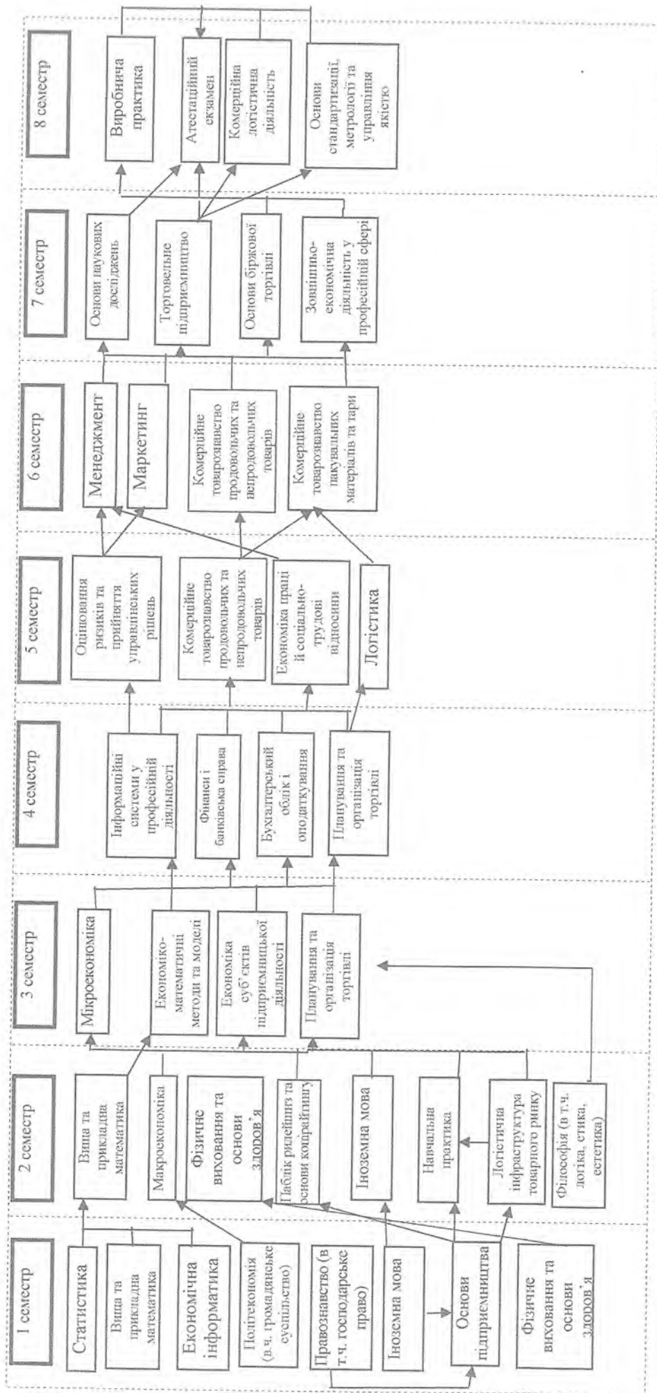
Рисунок 2.2.1 – Структурно-логічна схема
