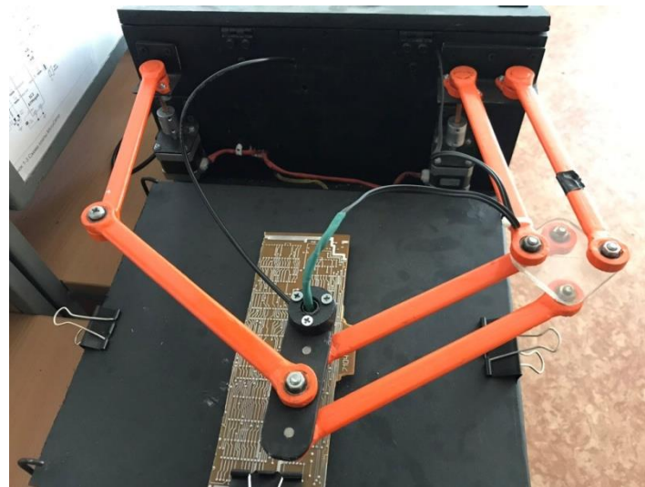
Рис. 1. Автоматичний паяльний маніпулятор
