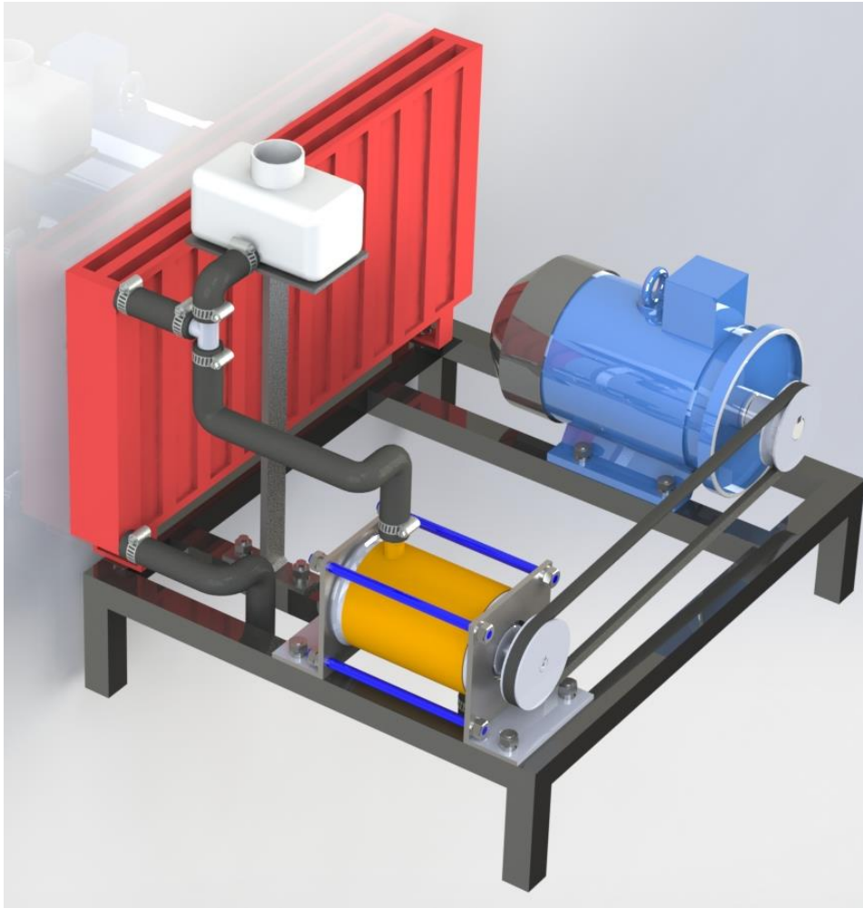
Рис. 1. Кавітаційний теплогенератор
