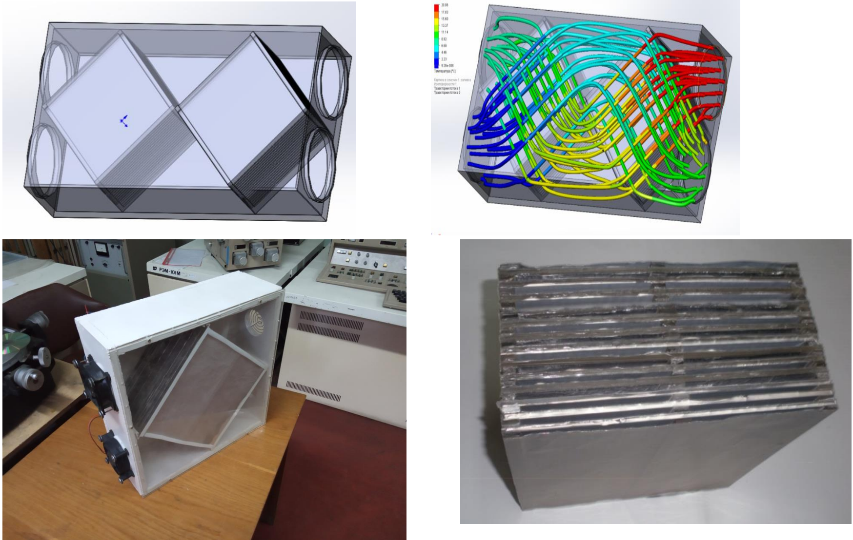
Рис. 1. Проектування пластинчатого рекуператора
