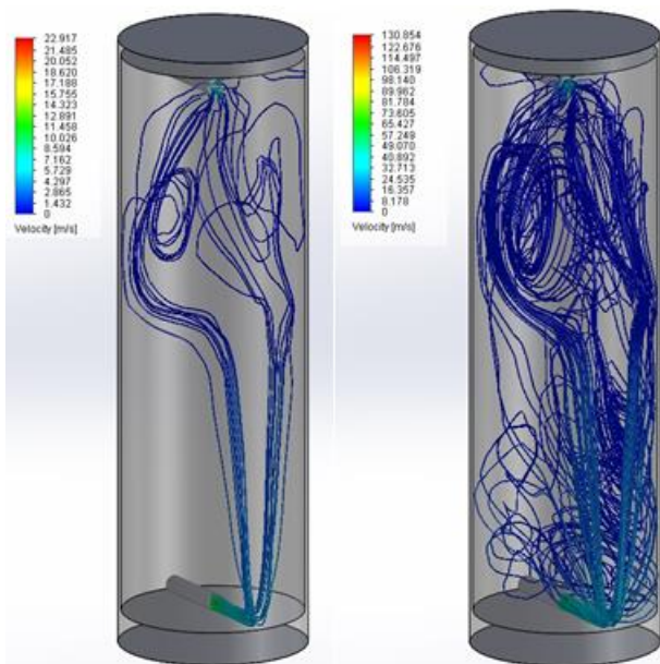
Рисунок 18 – Моделювання потоків течії в теплоаккумуляторі при його нагріванні на початку та через 1 годину
